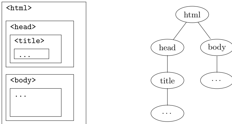
Bild 1.0: Block- und Baumdarstellung der Struktur eines HTML-Dokuments
